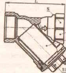
Рисунок 1. Фильтр осадочный ФО
