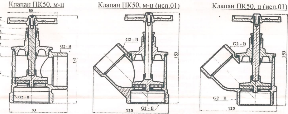
Рисунок 1. Клапан ПК50,
